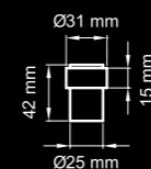
Bodentürstopper Erhöhung – EZ 215 G
