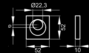
Schutzrosette – ESR 400Q KS
