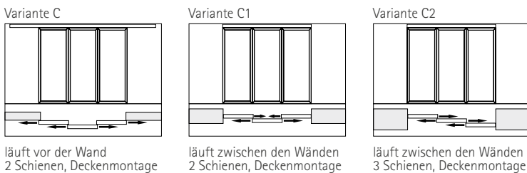
läuft vor der Wand 2 Schienen, Deckenmontage läuft zwischen den Wänden 2 Schienen, Deckenmontage
