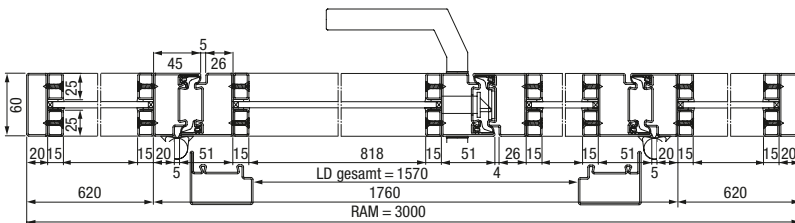
Horizontalschnitt 2-flügelige Stahl-Lofttür mit Seitenteilen und Oberlicht
