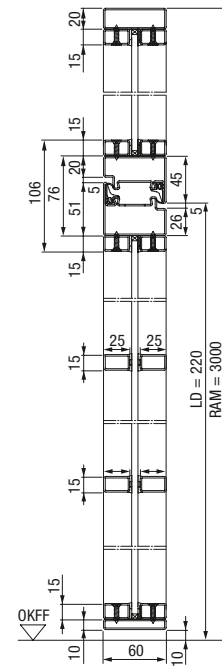
Vertikalschnitt 2-flügelige Stahl-Lofttür mit Seitenteilen und Oberlicht
