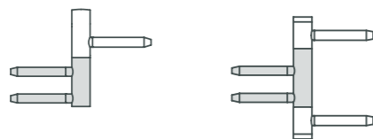
Band V 0020 Rahmenteil V 3400 WF Band V 0026 WF Rahmenteil V 4400 WF
