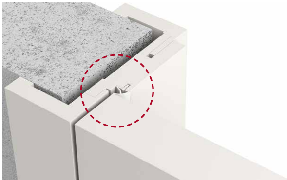
Stumpf – Das Türblatt ist stumpf und liegt in der Außenansicht auf der Dichtungsebene auf.
