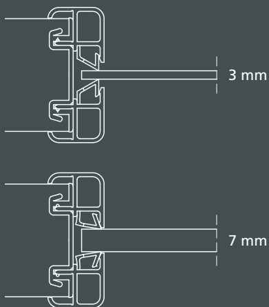
Längsseite fixieren
