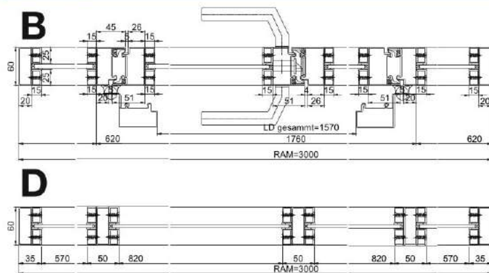
Horizontalschnitt
