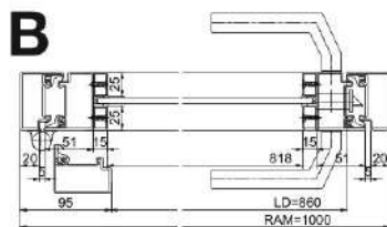
Ansicht 2-flüglige Tür
