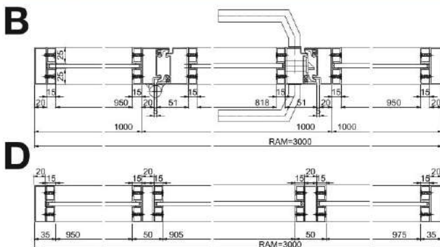
Horizontalschnitt
