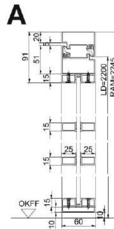
Vertikalschnitt
