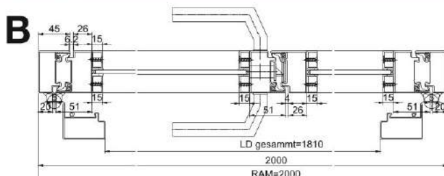
Horizontalschnitt
