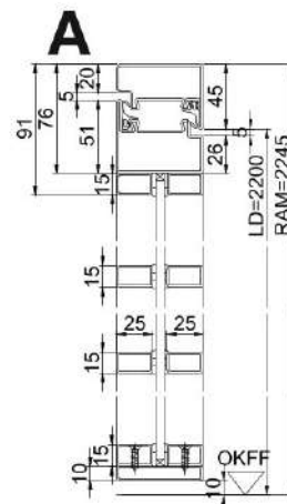
Vertikalschnitt
