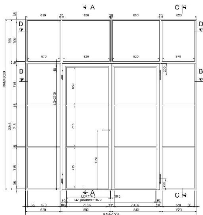
Vertikalschnitt
